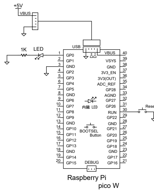
pico W Lチカ 電気回路図
